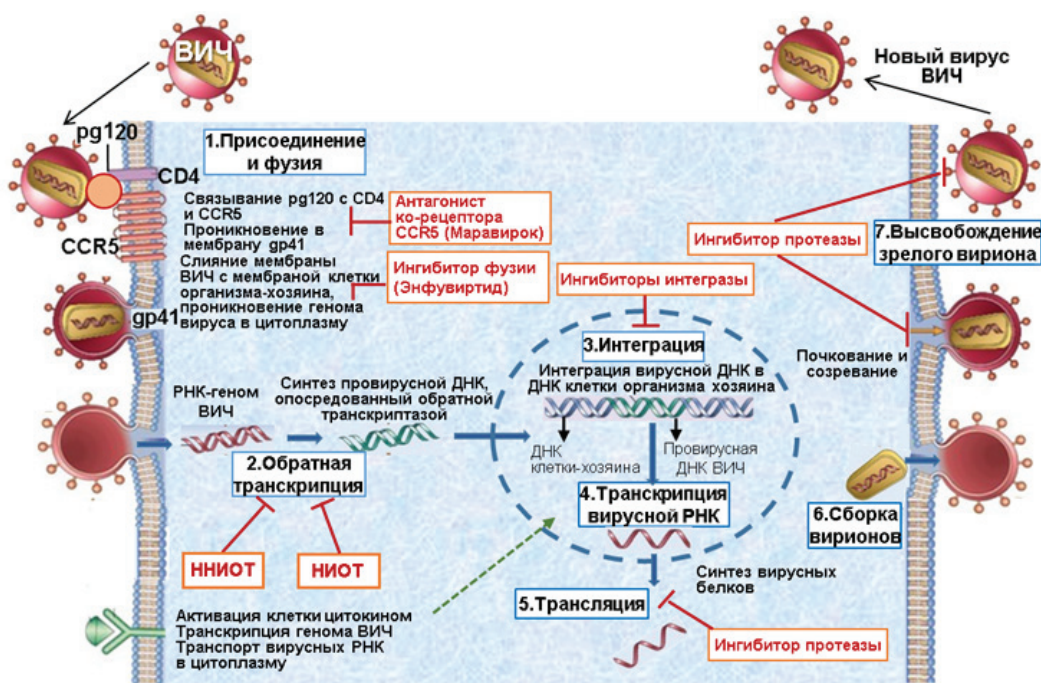
Рис. 1. Цикл репликации ВИЧ: точки приложения антиретровирусных препаратов
